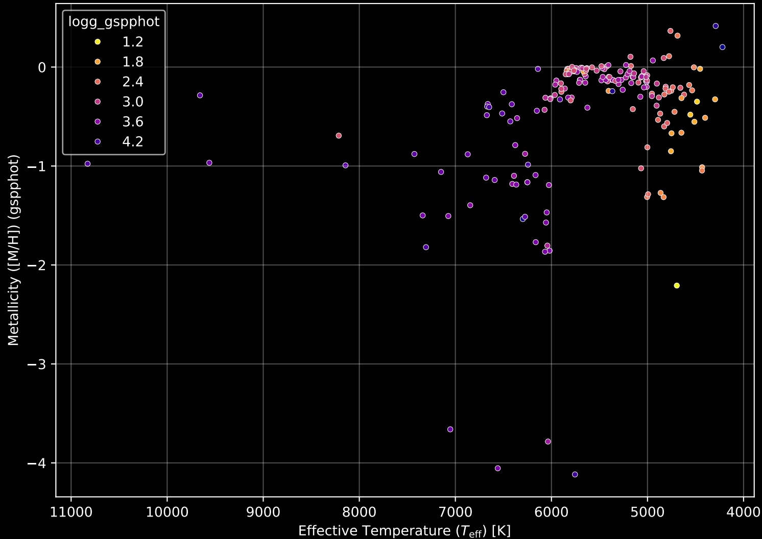
APOGEE DR17 Field: [M5] Stellar Population Parameters (n= 185)
